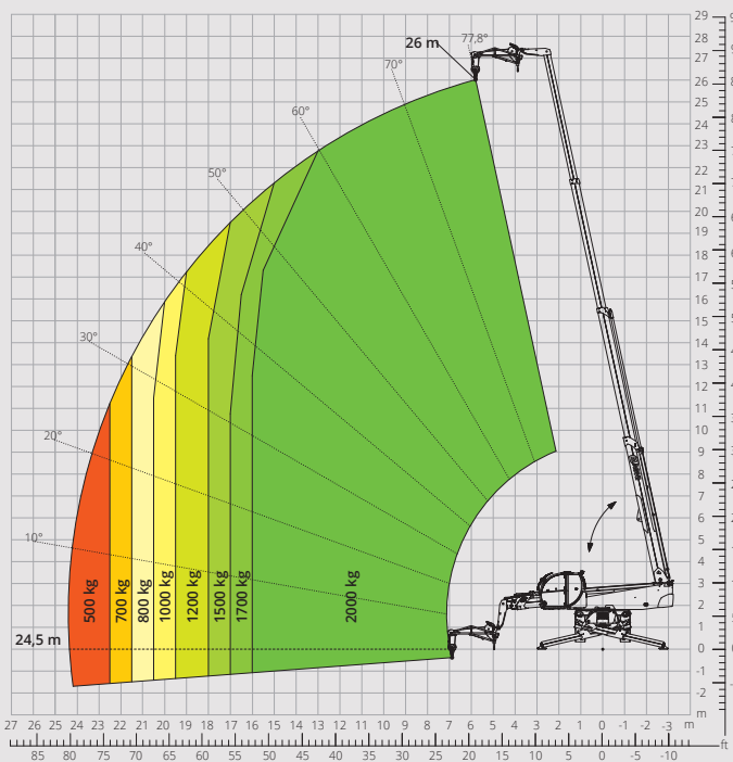
Diagram obciążeń z ŻURAWIEM Z WCIĄGARKĄ, 2.000 kg ATT - 04 - 015
