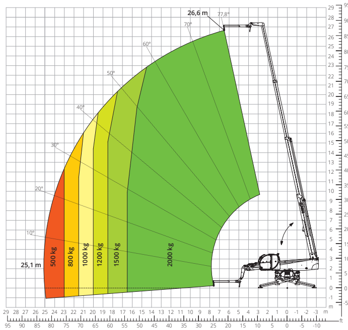
Diagram obciążeń z PLATFORMĄ OBROTOWĄ ROZSUWANĄ, 1.000 kg ATT - 01 - 016
