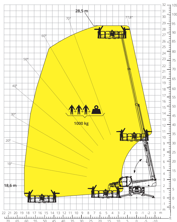
Diagram obciążeń z PLATFORMĄ OBROTOWĄ ROZSUWANĄ, 1.000 kg ATT - 01 - 016
