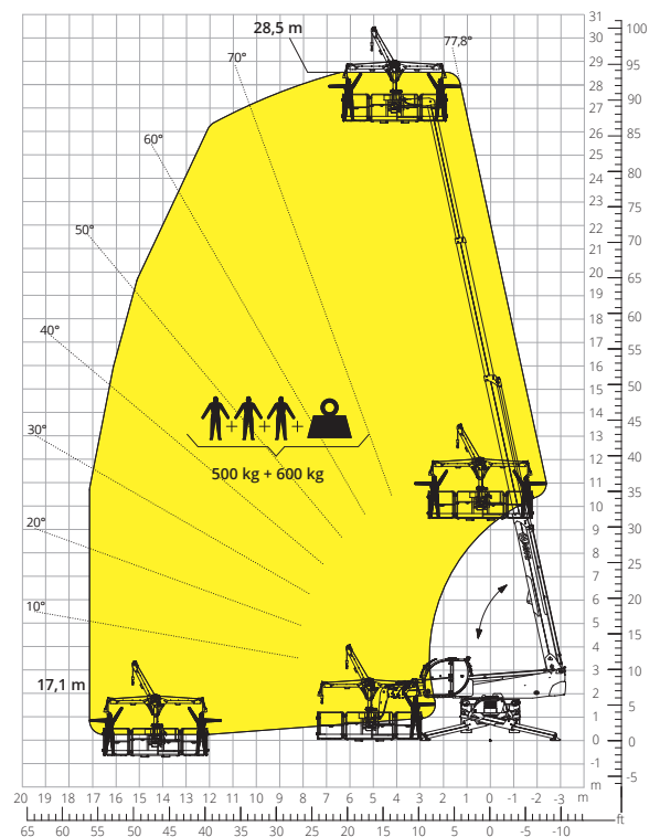
Diagram obciążeń z PLATFORMĄ, 500 kg, Z WCIĄGARKĄ, 600 kg ATT - 01 - 026
