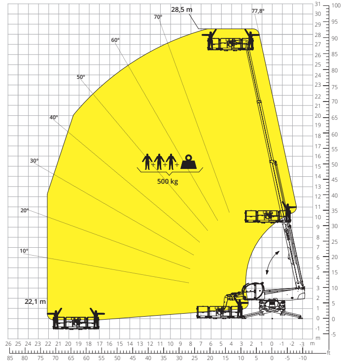
Diagram obciążeń z PLATFORMĄ, 500 kg, Z WCIĄGARKĄ, 600 kg ATT - 01 - 026
