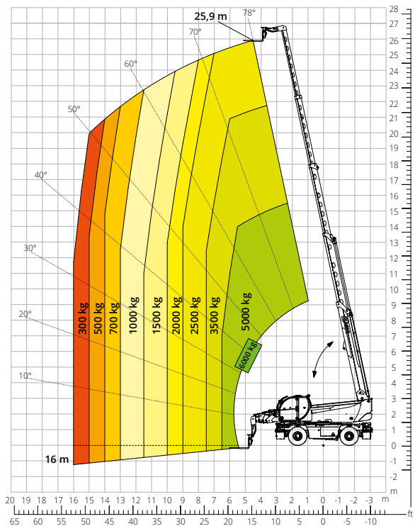
Diagramma portate FRONTALE SU PNEUMATICI ATT-03-004
