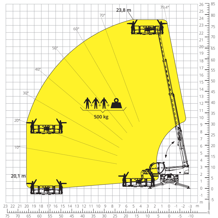
Diagram obciążeń z PLATFORMĄ, 500 kg, Z WCIĄGARKĄ, 600 kg ATT - 01 - 026
